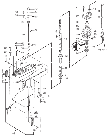
Fig. 11A GEAR CASE (DRIVE SHAFT) ギヤケース (ドライブシャフト)
