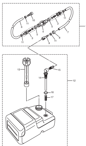
Fig. 25 FUEL TANK フエルトンク
