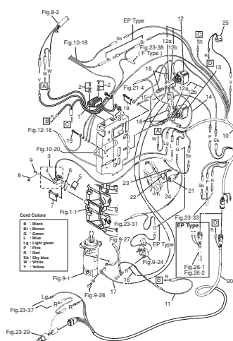
Fig. 11 ELECTRIC PARTS (DIAGRAM) エレクトリックパーツ (ダイヤグラム)
