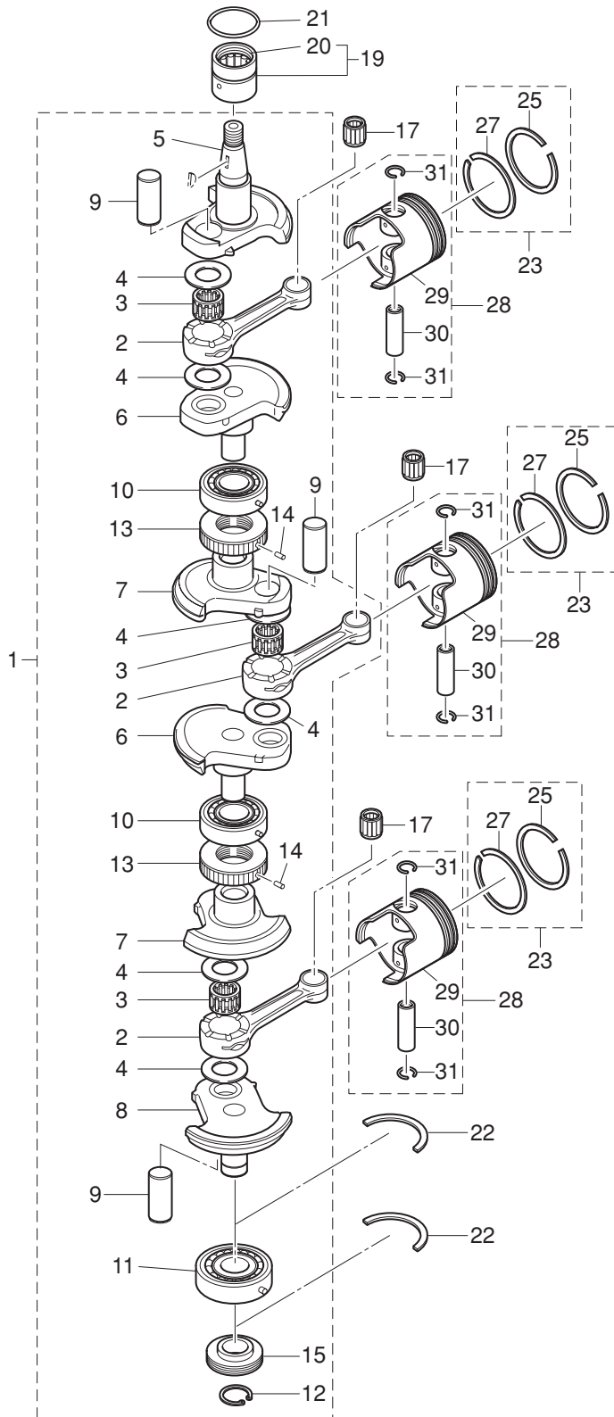
PISTON・CRANK SHAFT ピストン・クランクシャフト
