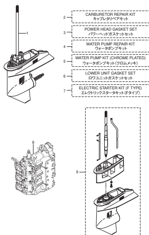
Fig. 33 ASSEMBLY · KIT PARTS アセンブリ・キットパーツ
