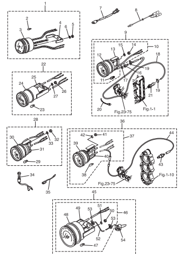
Fig. 32 OPTIONAL PARTS (5) オプションパーツ (5)
