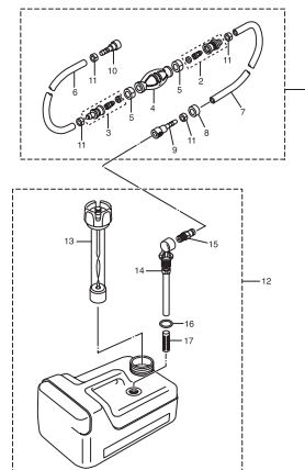
Fig. 18 OPTIONAL PARTS (ACCESSORIES) オプションパーツ (アクセサリ)
