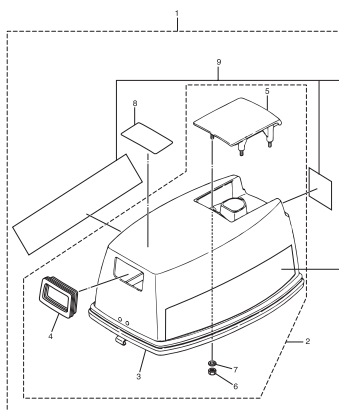
Fig. 14 TOP COWL トップカウル
